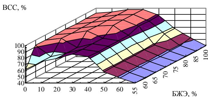
Рис. 1. Изменение ВСС и ВУС фарша вареных колбас в зависимости от уровня использования БЖЭ
