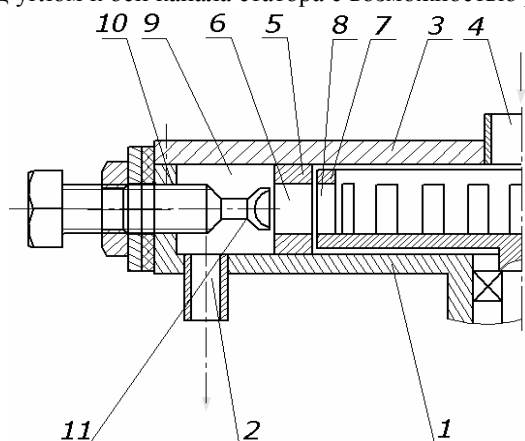
Рис. 1. Принципиальная схема роторного аппарата
