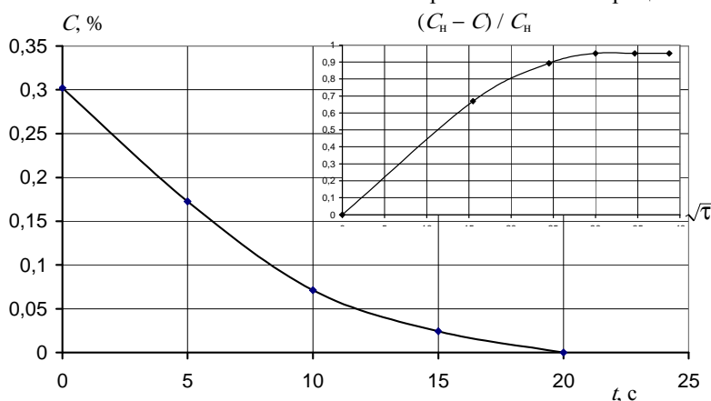
Рис. 1. Кинетика изменения среднего влагосодержания образца ПЭНД-композита с массовой долей УНМ 0,2 мас. ч.
