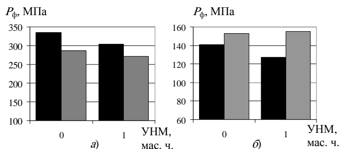
Рис. 1. Диаграмма изменения давления ТФЭ наноккомпозитов на основе:
