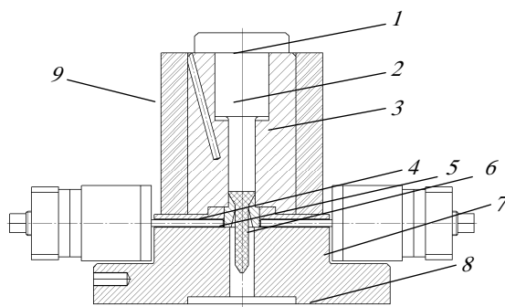
Рис. 2. Экспериментальная ячейка высокого давления с ультразвуковыми излучателями:
