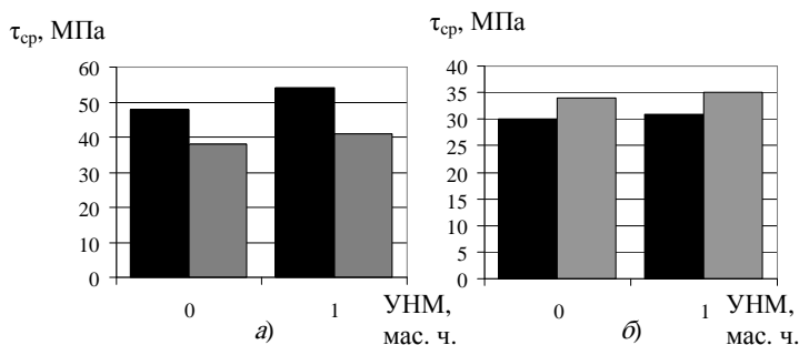
Рис. 2. Диаграмма изменения прочности в условиях среза наноккомпозитов на основе:
