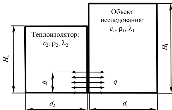
Рис. 2. Тепловая схема
