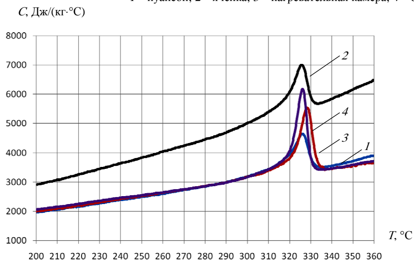
Рис. 2. Термограммы фторопласта и композитов на его основе, полученные в цикле нагревания:
