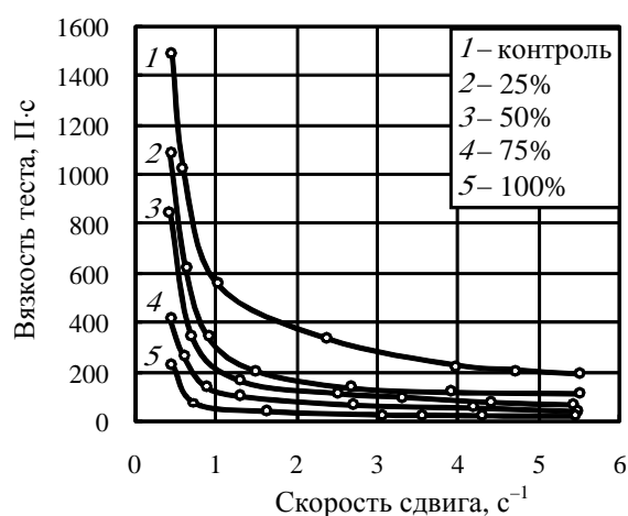
Зависимость эффективной вязкости теста от скорости сдвига при различной дозировке БЗП, % к массе сухих веществ Влияние дозировки БЗП на качество овсяного печенья
