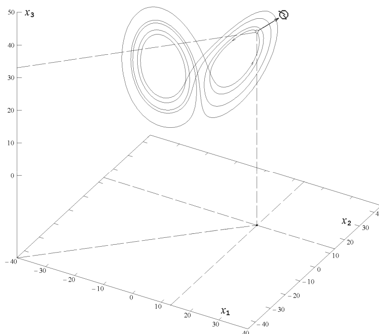
Рис. 2. Дуга траектории системы Лоренца, построенная на отрезке времени [0; 6,827] , для начальной точки с координатами (13,41265629; 13,46430003; 33,46156416) . Стрелкой отмечено возвращение в \epsilon -окрестность ( \epsilon = 0,11 )
