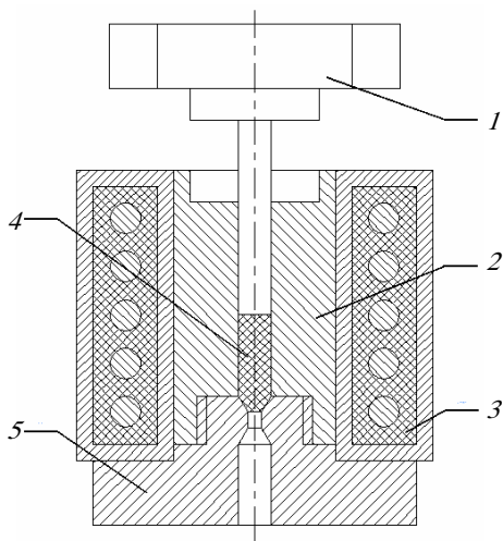
Рис. 1. Ячейка высокого давления типа капиллярного вискозиметра для реализации плунжерной твердофазной экструзии: 1 – пуансон; 2 – ячейка; 3 – нагревательная камера; 4 – образец; 5 – фильера
