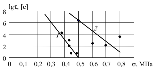
Рис. 2. Влияние армирования пенополистирола ПСБС-М 35 на долговечность при поперечном изгибе при температуре 20°C: 1 – неармированная конструкция; 2 – армированная конструкция
