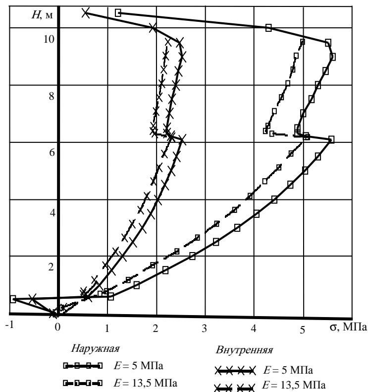
Рис. 2. Зависимости изменения напряжений в полках стоек от координат сечений рамы при податливом основании
