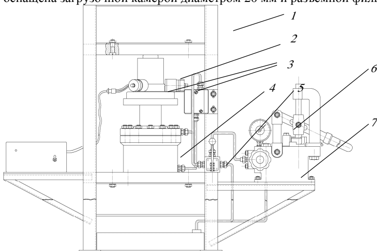
Рис. 1. Установка для твердофазной экструзии полимеров с использованием ультразвуковых излучателей:
