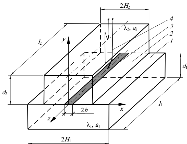
Рис. 1. Измерительная схема метода с линейным источником тепла:
