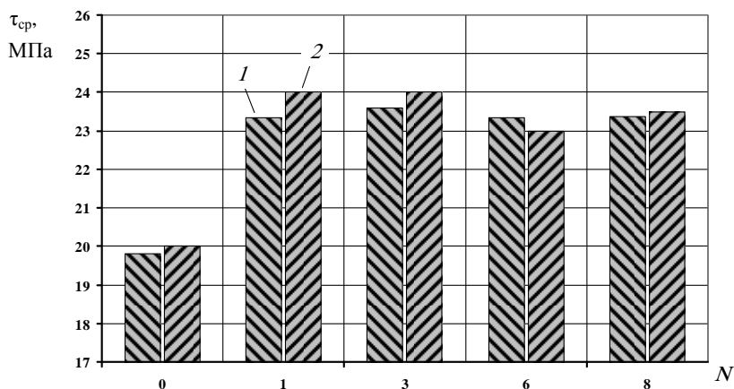
Рис. 2. Диаграмма изменения прочности в условиях срезающих напряжений \tau_{ср} в зависимости от числа циклов деформирования N в ячейке РКМУТФЭ: ПЭВП + 1 мас. ч. УНМ; T_{экс} = 295 К; 1 – образцы получены традиционным способом с последующей обработкой в режиме РКМУТФЭ; 2 – образцы получены в смесителе Haake Polydrive с последующей обработкой в режиме РКМУТФЭ
