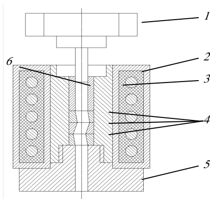
Рис. 1. Схема экспериментальной ячейки высокого давления для реализации равноканальной многоугловой твердофазной экструзии:
