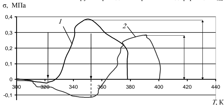
Рис. 3. Диаграмма изометрического нагрева образцов ПЭВП, полученных: 1 – традиционным методом; 2 – в смесителе Haake Polydrive, с последующей обработкой давлением в режиме ТФЭ
