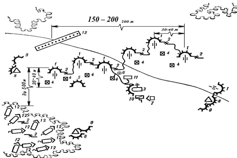
Рис. 13.2.2 Схема инженерного оборудования огневой позиции батареи буксируемых орудий (вариант): 1 – окоп для орудия; 2 – перекрытая щель; 3 – окоп для машины старшего офицера батареи 1В110; 4 – погребок для боеприпасов; 5 – открытое сооружение для командира огневой взвода; 6 – пункт водоснабжения; 7 – укрытие для агрегата АБ-1; 8 – открытое сооружение для наблюдательного поста; 9 – окоп для самообороны; 10 – блиндаж; 11 – убежище; 12 – укрытие для тягача и других транспортных средств; 13 – противотанковое минное поле
