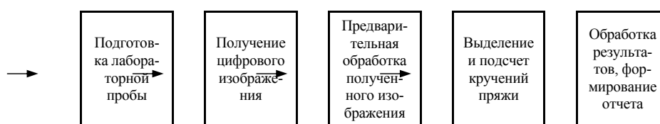
Рис. P.1 Последовательность операций компьютерного метода измерения показателей скрученности пряжи
