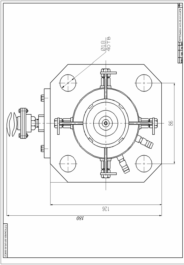
Рис. Г.6 Сборочный чертеж головки прямоугольной (лист 2)
