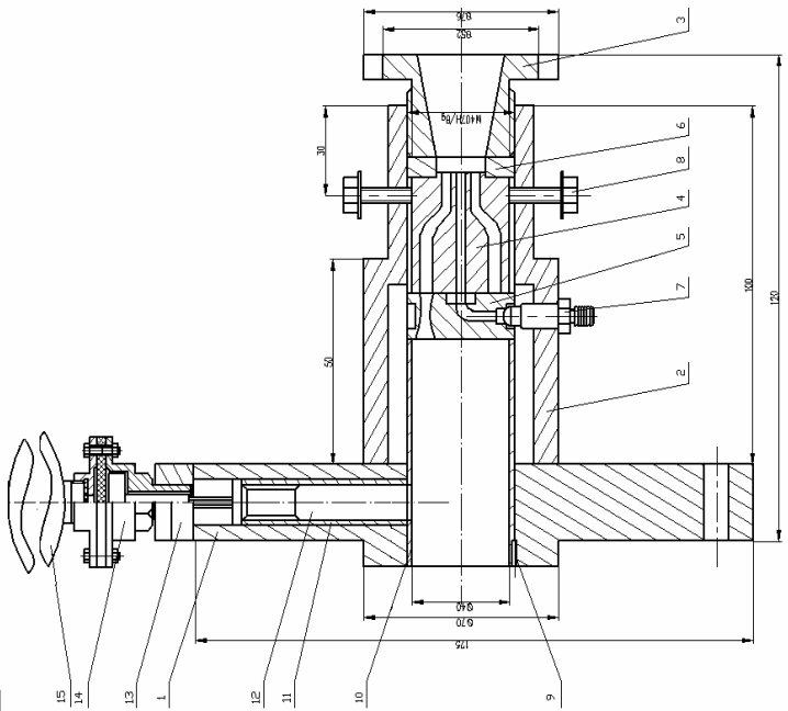
Рис. Г.5 Сборочный чертеж головки прямоугольной (лист 1)
