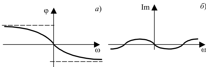
Рис. 4.7 Свойство нечетности частотных характеристик: а – ФЧХ; б – МЧХ
