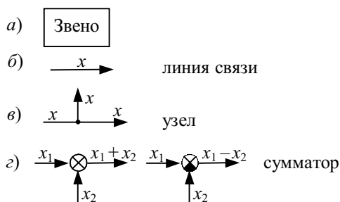
Рис. 5.27 Условные обозначения элементов структурной схемы
