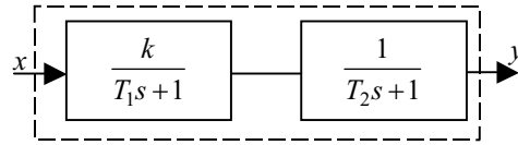
Рис. 5.20 Структурная схема аperiodического звена второго порядка
