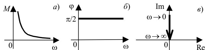
Рис. 5.54 Частотные характеристики И-закона регулирования: a – АЧХ; б – ФЧХ; в – АФХ
