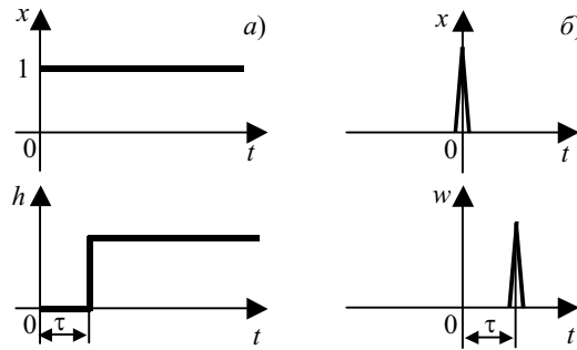
Рис. 5.13 Переходные характеристики звена чистого запаздывания: а – переходная функция; б – весовая функция
