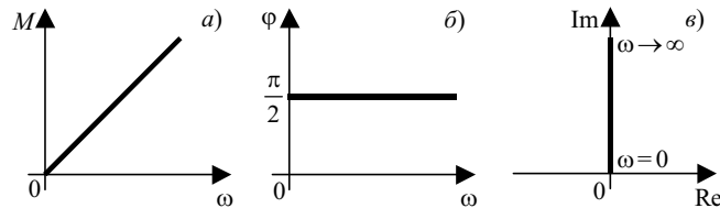
Рис. 5.5 Частотные характеристики идеального дифференцирующего звена: a – АЧХ; б – ФЧХ; в – АФХ
