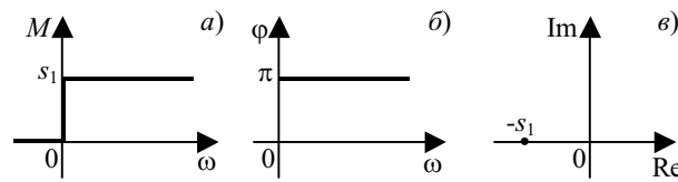
Рис. 5.51 Частотные характеристики П-регулятора: а – АЧХ; б – ФЧХ; в – АФХ
