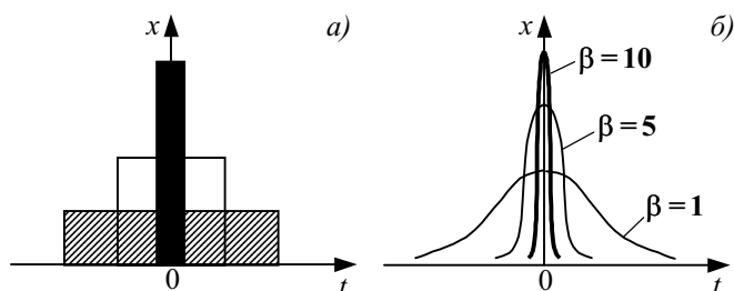
Рис. 2.7 Представление дельта-функции: а – прямоугольный импульс; б – \delta(\beta, t) -функция
