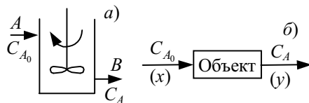
Рис. 3.4 Химический реактор: a – принципиальная схема; б – структурная схема
