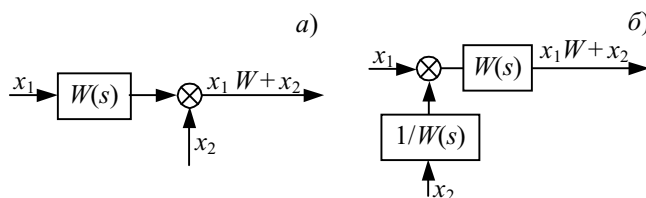
Рис. 5.43 Перенос звена через сумматор: a – до преобразования; б – после преобразования
