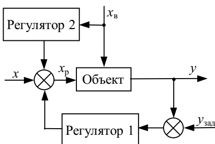
Рис. 1.13 Структурная схема АСР
