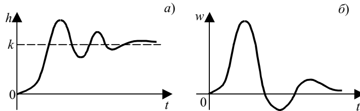
Рис. 5.24 Переходные характеристики колебательного звена: а – переходная функция; б – весовая функция
