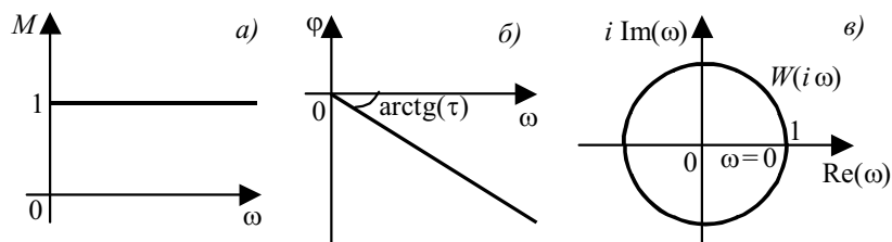
Рис. 5.12 Частотные характеристики звена чистого запаздывания: а – АЧХ; б – ФЧХ; в – АФХ
