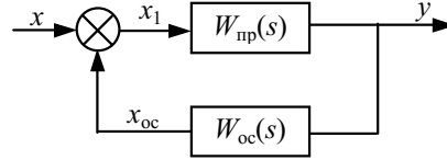
Рис. 5.33 Соединение с обратной связью
