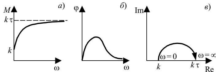
Рис. 5.16 Частотные характеристики инерционно-форсирующего звена для \tau > 1 :
