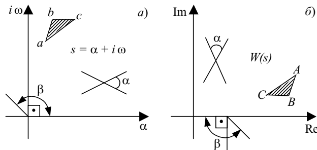
Рис. 4.4 Конформное отображение
