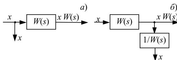
Рис. 5.40 Перенос узла через звено: a – до преобразования; б – после преобразования
