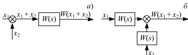
Рис. 5.42 Перенос сумматора через звено: a – до преобразования; б – после преобразования
