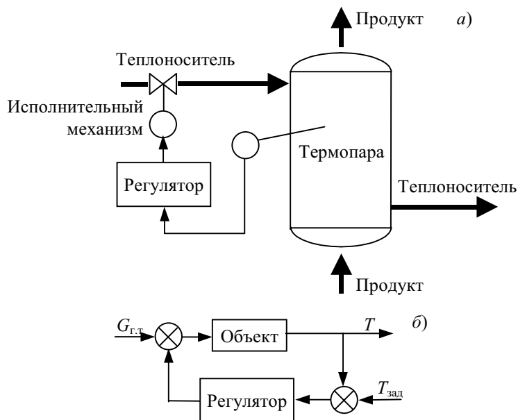
Рис. 1.9 Система регулирования температуры продукта в теплообменнике:
