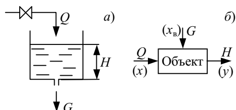
Рис. 3.2 Гидравлическая емкость:
