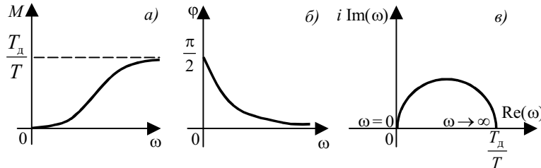
Рис. 5.7 Частотные характеристики реального дифференцирующего звена: a – АЧХ; b – ФЧХ; c – АФХ
