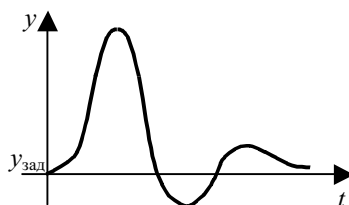
Рис. 5.56 Переходный процесс в АРС с И-регулятором
