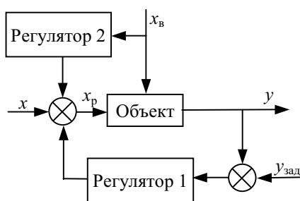
Рис. 1.8 Структурная схема комбинированной АСР
