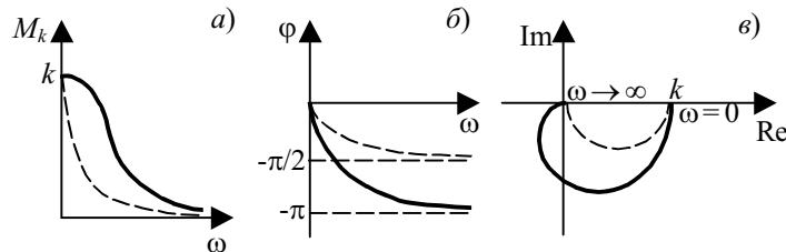
Рис. 5.21 Частотные характеристики аperiodического звена второго порядка:
