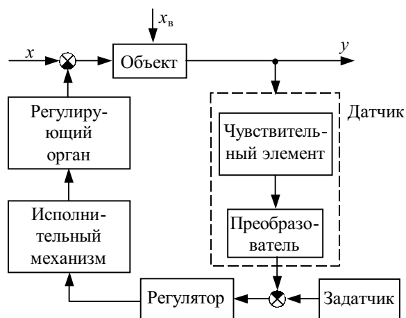
Рис. 1.11 Структурная схема АСР
