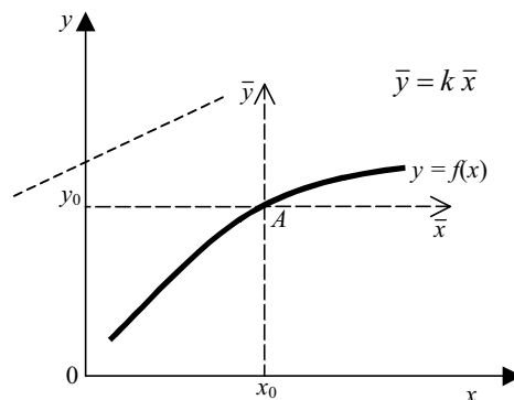
Рис. 3.6 Линеаризация нелинейной статической характеристики
