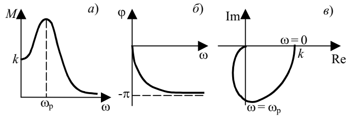
Рис. 5.23 Частотные характеристики колебательного звена: а – АЧХ; б – ФЧХ; в – АФХ
