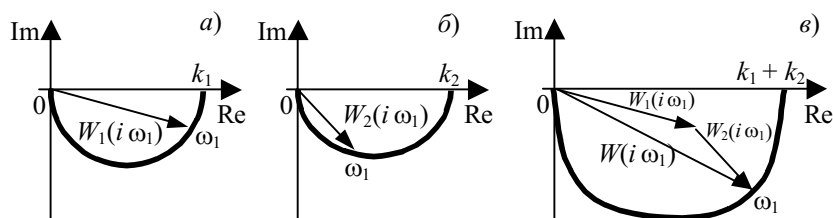
Рис. 5.29 Построение АФХ параллельного соединения: a – АФХ первого звена; б – АФХ второго звена; в – АФХ параллельного соединения первого и второго звеньев
