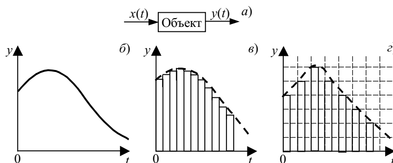
Рис. 2.4 Виды математических представлений сигналов:
