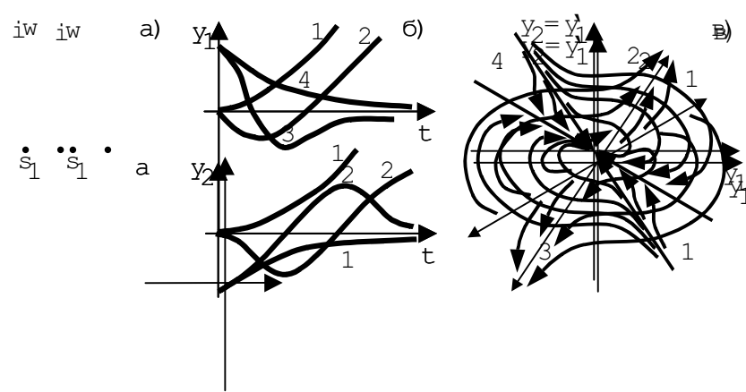
Рис. 6.10 Фазовый портрет типа устойчивый узел:
