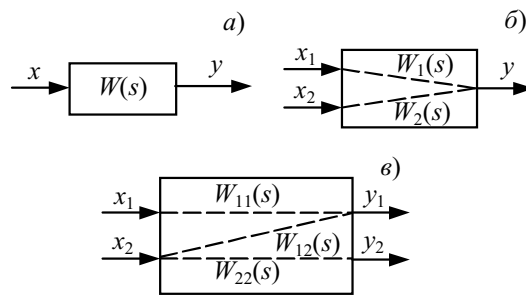
Рис. 3.13 Примеры различных объектов: a – с одним входом и одним выходом; б – двумя входами и одним выходом; в – двумя входами и двумя выходами
