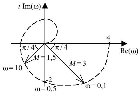
Рис. 4.11 Годограф АФХ
