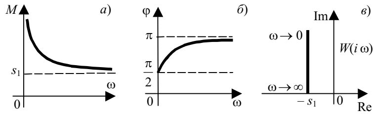
Рис. 5.62 Частотные характеристики ПИ-регулятора: a – АЧХ; б – ФЧХ; в – АФХ
