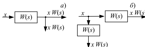
Рис. 5.41 Перенос звена через узел: a – до преобразования; б – после преобразования
