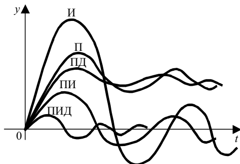
Рис. 5.67 Переходные процессы в АСР с различными законами регулирования
