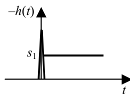
Рис. 5.60 Переходная функция ПД-регулятора
