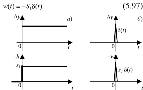
Рис. 5.52 Переходные характеристики П-регулятора: а – переходная функция; б – весовая функция
