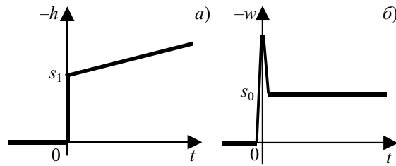
Рис. 5.63 Переходные характеристики: a – переходная функция; б – весовая функция
