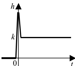
Рис. 5.10 Переходная функция форсирующего звена
