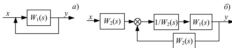
Рис. 5.47 Внесение элемента в обратную связь: a – до преобразования; б – после преобразования
