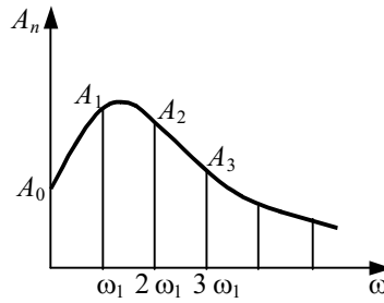
Рис. 2.3 Спектр периодического сигнала
