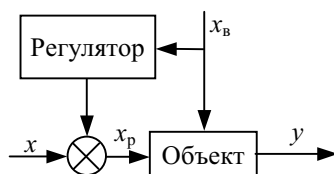
Рис. 1.7 Структурная схема регулирования по возмущению
