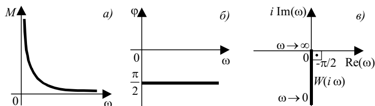
Рис. 5.3 Частотные характеристики интегрирующего звена: a – АЧХ; б – ФЧХ; в – АФХ
