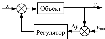
Рис. 1.6 Структурная схема регулирования по отклонению
