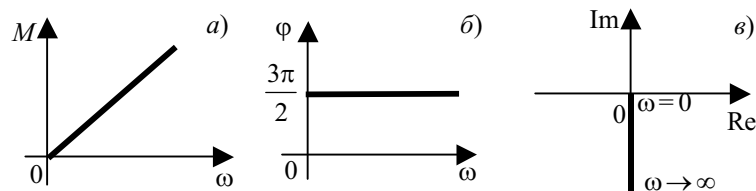
Рис. 5.57 Частотные характеристики Д-закона регулирования: а – АЧХ; б – ФЧХ; в – АФХ
