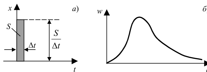
Рис. 3.11 Переходная характеристика химического реактора:
