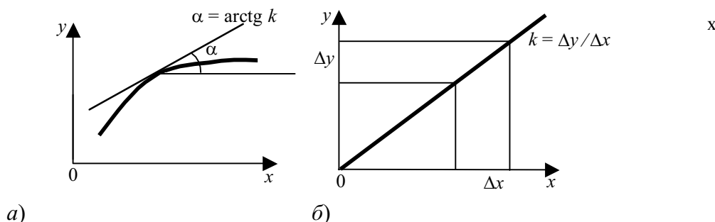
Рис. 3.1 Статическая характеристика объектов: а – нелинейного; б – линейного
