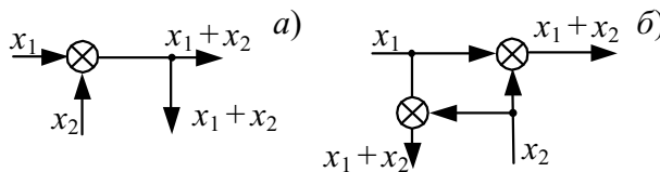
Рис. 5.39 Перенос сумматора через звено: a – до преобразования; б – после преобразования
