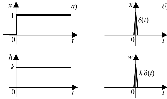
Рис. 5.2 Графики временных характеристик усилительного звена: a – переходная функция; б – весовая функция
