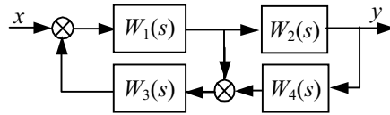
Рис. 5.50 Структурная схема технологического объекта
