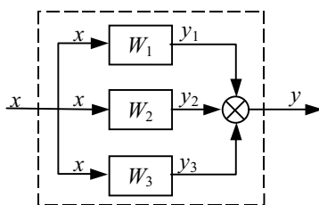
Рис. 5.28 Параллельное соединение звеньев
