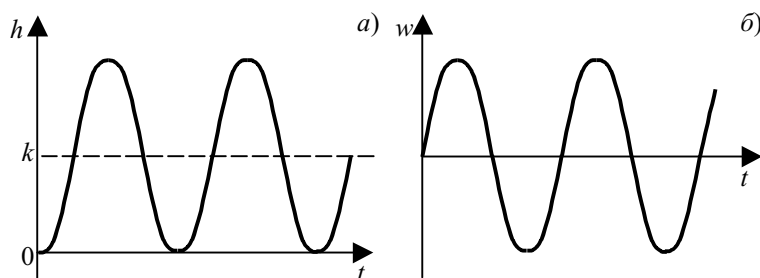
Рис. 5.26 Функции консервативного звена: а – переходная; б – весовая
