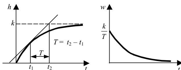
Рис. 5.15 Переходные характеристики апериодического звена первого порядка:
