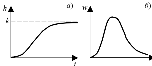
Рис. 5.22 Переходные характеристики аperiodического звена второго порядка:
