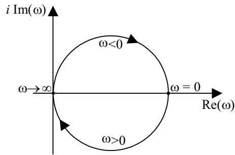
Рис. 4.8 Годограф АФХ
