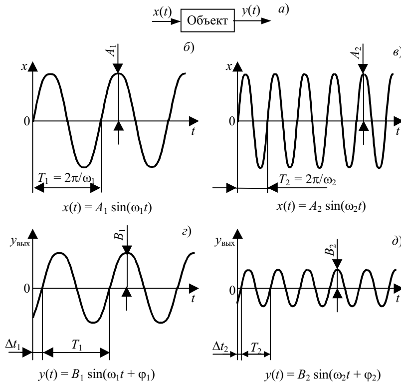
Рис. 4.10 Экспериментальное определение частотных характеристик: a – объект; б – входной сигнал частоты \omega_1 ; в – входной сигнал частоты \omega_2 ; г – выходной сигнал частоты \omega_1 ; д – выходной сигнал частоты \omega_2
