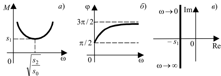
Рис. 5.65 Частотные характеристики ПИД-регулятора: a – АЧХ; b – ФЧХ; c – АФХ
