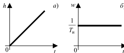
Рис. 5.4 Переходные характеристики интегрирующего звена: а – переходная функция; б – весовая функция
