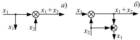
Рис. 5.38 Перенос узла через сумматор: a – до преобразования; б – после преобразования
