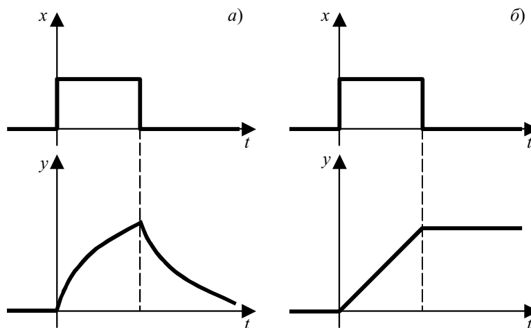
Рис. 6.2 Переходные процессы при импульсном возмущении: a – апериодическое звено первого порядка; b – интегральное
